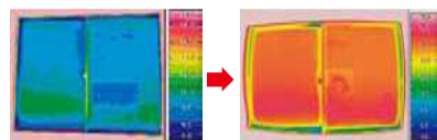
<外窓のみ> 青色部分で約5℃ <外窓+インプラス> 橙色部分で約25℃
